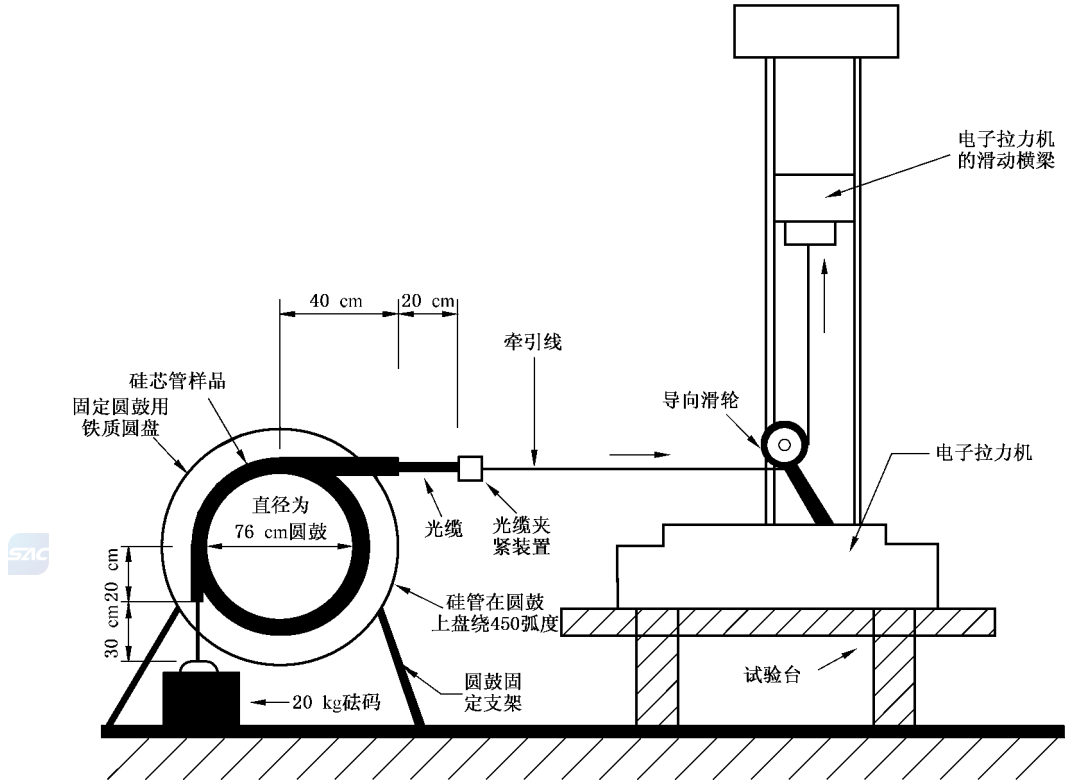
图 D.1 圆鼓法测定摩擦系数试验示意图
